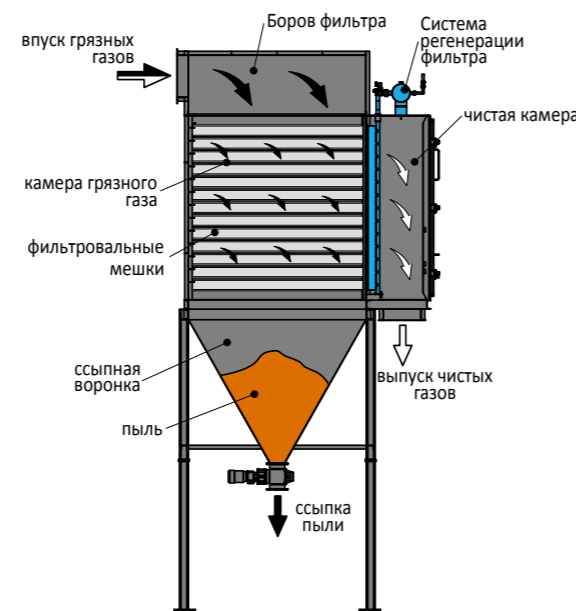
Функциональная схема горизонтального мешочного фильтра
